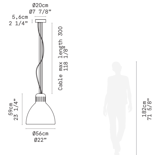
JJ GREAT - PENDANT
